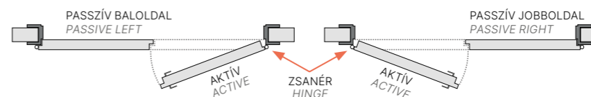
KÉTSZÁRNYÚ AJTÓ, JOBOS DOUBLE LEAF DOOR, RIGHT
